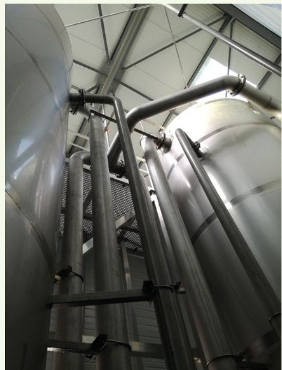
Station de traitement de Frangy-en-Bresse Filtres à charbon actif (SME de la Seillette)
